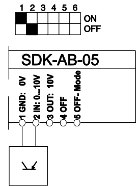
Ansteuerung mit Sinkstromquelle (LV-L2EVG)
